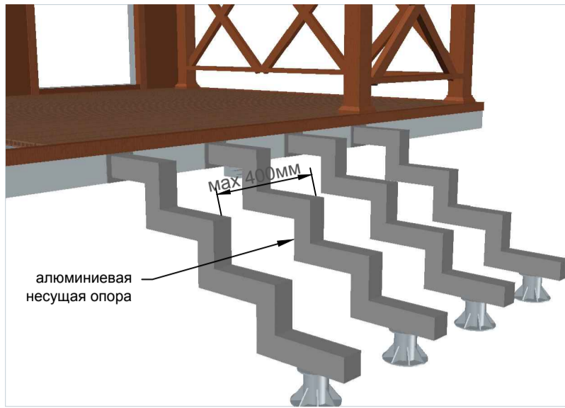
МОНТАЖ ЛЕСТНИЦЫ
