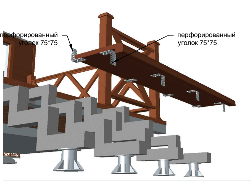
МОНТАЖ СТУПЕНЕЙ
