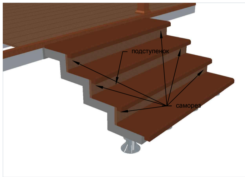
МОНТАЖ ПОДСТУПЕНИЙ
